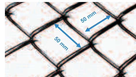
Drahtstärke 3,10 mm Kunststoff ummantelt
