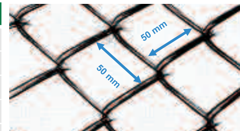
Drahtstärke 2,20 mm dick verzinkt und 2,80 mm Kunststoff ummantelt
